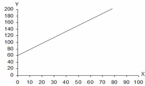
Grafik 1. Regresi Linear Sederhana \hat{Y} = 60,07 + 1,81X
