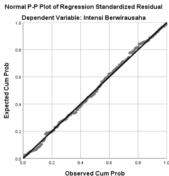
Gambar 2. Uji Normalitas
