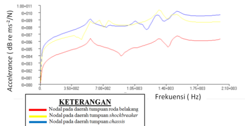
Gambar 4.86 Grafik Accelerance Modulus Model Modifikasi
