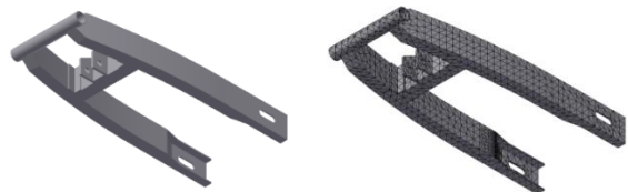
Gambar 9.1 Geometri dan Meshing Model Modifikasi
