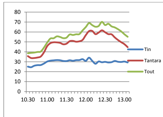
Gambar 10. Hasil pengukuran temperatur terhadap waktu hari ketiga.
