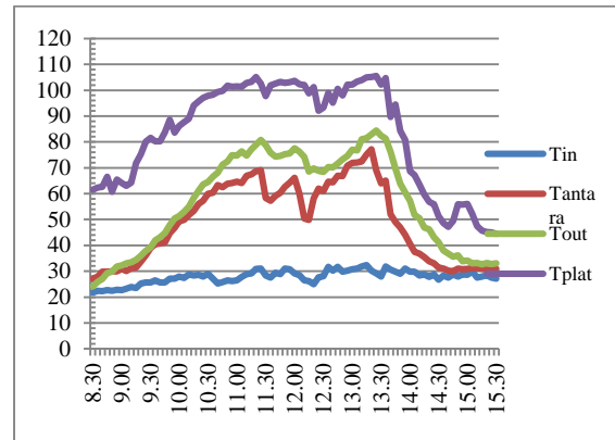
Gambar 8. Hasil pengukuran temperatur terhadap waktu hari kedua. Sinar matahari mulai terhalang awan mulai pukul 13.30.
