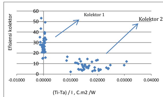
Gambar 9. Efisiensi kolektor.
