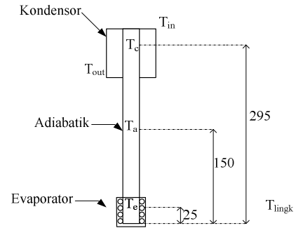
Gambar 7. Pemasangan termokopel pada pipa kalor (mm)
