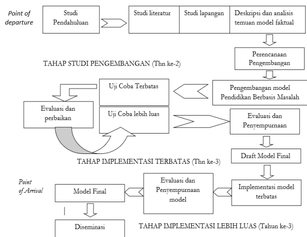
Gambar 1. Langkah-langkah penelitian
