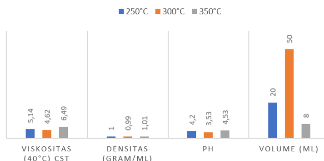
Gambar 1. Grafik hasil penelitian dengan variasi suhu pirolisis
