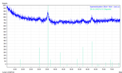
Gambar 6. Hasil Pola difraksi \text{Fe}_3\text{O}_4
