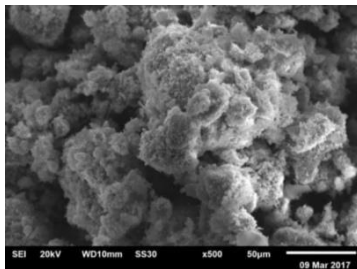
Gambar 4. Hasil SEM \text{Fe}_3\text{O}_4
