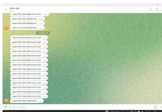
Gambar 8 Notifikasi Telegram
