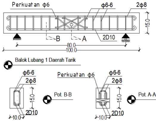
Gambar 4. Balok Belulang 1 Daerah Tarik (BBTA1)
