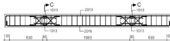
Gambar 11. Balok Berlubang Persegi Ganda
