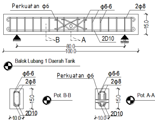
Gambar 5. Balok Berlulang 2 di Daerah Tarik (BBTA2)
