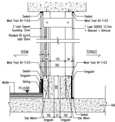
Gambar 3. Detail Drywall untuk Dinding Luar
