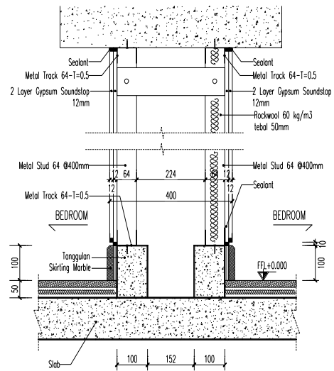
Gambar 4. Detail Dinding Penyekat Ruangan
