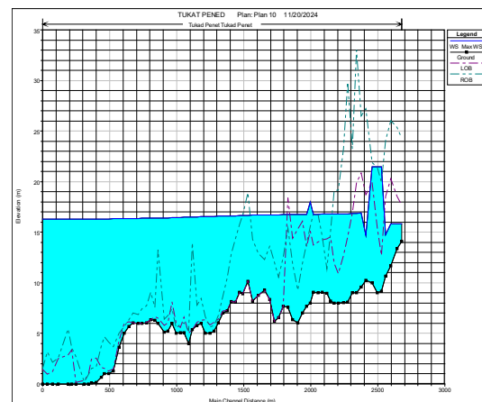
Gambar 7. Profil Muka Air Unsteady Flow
