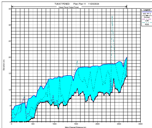
Gambar 5. Profil Muka Air Steady Flow
