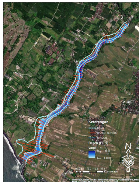
Gambar 4. Hasil Simulasi 1D Menggunakan Steady Flow
