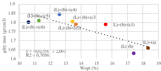
Gambar 4. Hubungan Nilai \gamma_{dry} Max dengan W_{opt} Variasi Campuran Tanah Lunak, Pasir, Air Tawar, dan Air Laut
