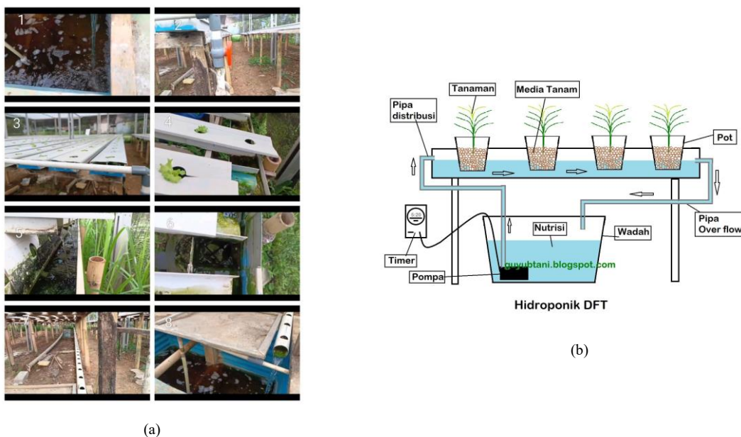
Gambar 2 (a) dan (b). Tahapan-tahapan prinsip kerja dalam sistem DFT di RHTB. (Sumber: https://guyubtani.blogspot.com/2016/05/cara-bertanam-hidroponik-dft-deep-flow-technique.html dan Penuli 2025)
