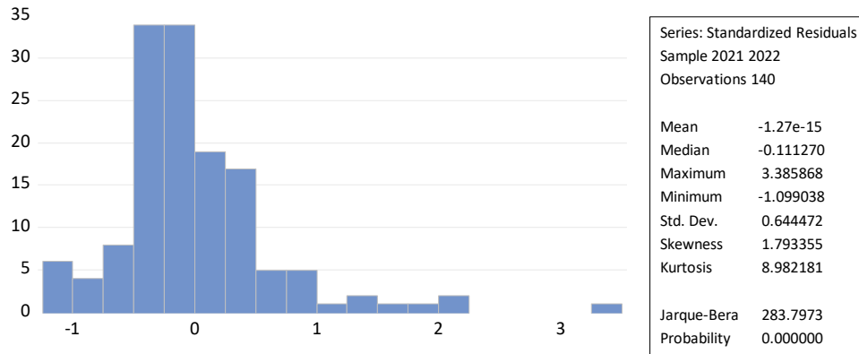
Gambar 2. Uji Normalitas – sebelum outlier
