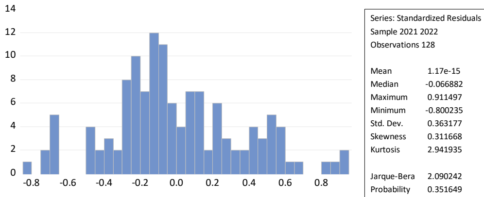
Gambar 3. Uji Normalitas – sesudah outlier
